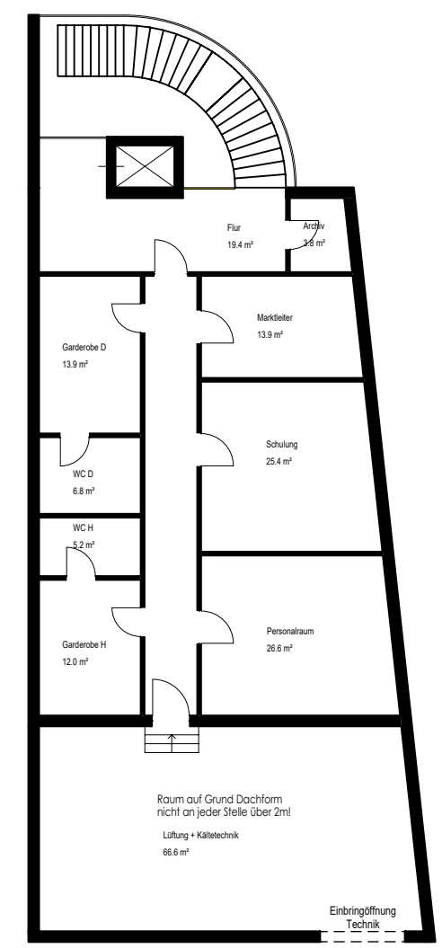
1. Obergeschoss
